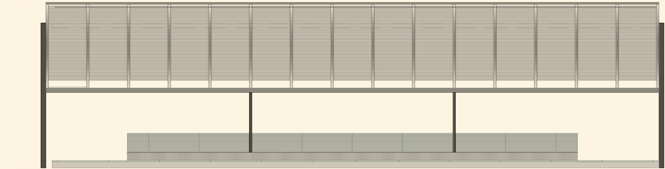
ALZADO FRONTAL PRINCIPAL - FACHADA A
